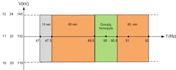
Σχεδιάγραμμα 1: Υποχρεωτική Δυνατότητα Λειτουργίας Αιολικών Πάρκων (εντός του εύρους Τάσης κανονικής λειτουργίας του Ηλεκτρικού Συστήματος) σε συνάρτηση με τη Συχνότητα.
