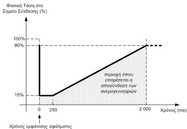
Σχεδιάγραμμα 4: Καμπύλη Τάσης για Αδιάλειπτη Λειτουργία ανεμογεννητριών.
